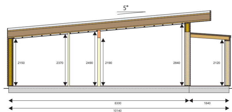
Snitt
